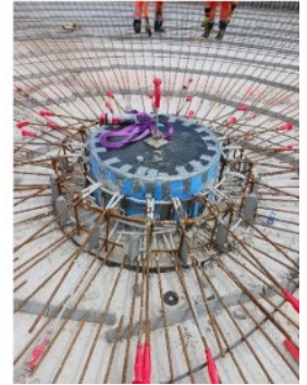
16 avril : Ferrailage radier du bassin biologique, radier fosse centrale du clarificateur, pose des conduites sous l'ouvrage, pré fouille et béton de propreté du bassin d'orage.
